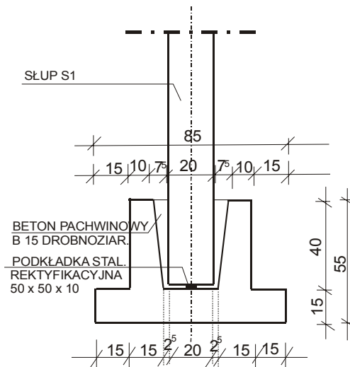
PRZEKRÓJ A-A sk. 1:20
